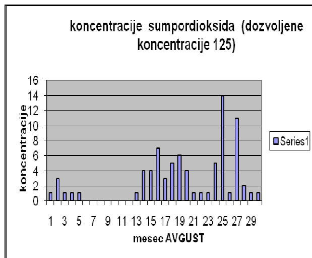
График 1 – Приказ добијених резултата испитивања испитивања за параметар сумпор-диоксид у односу на ГВ
