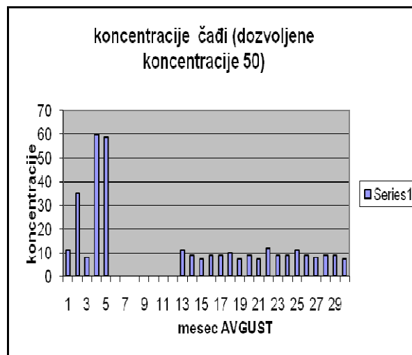
График 2 – Приказ добијених резултата за параметар чађи у односу на ГВ
